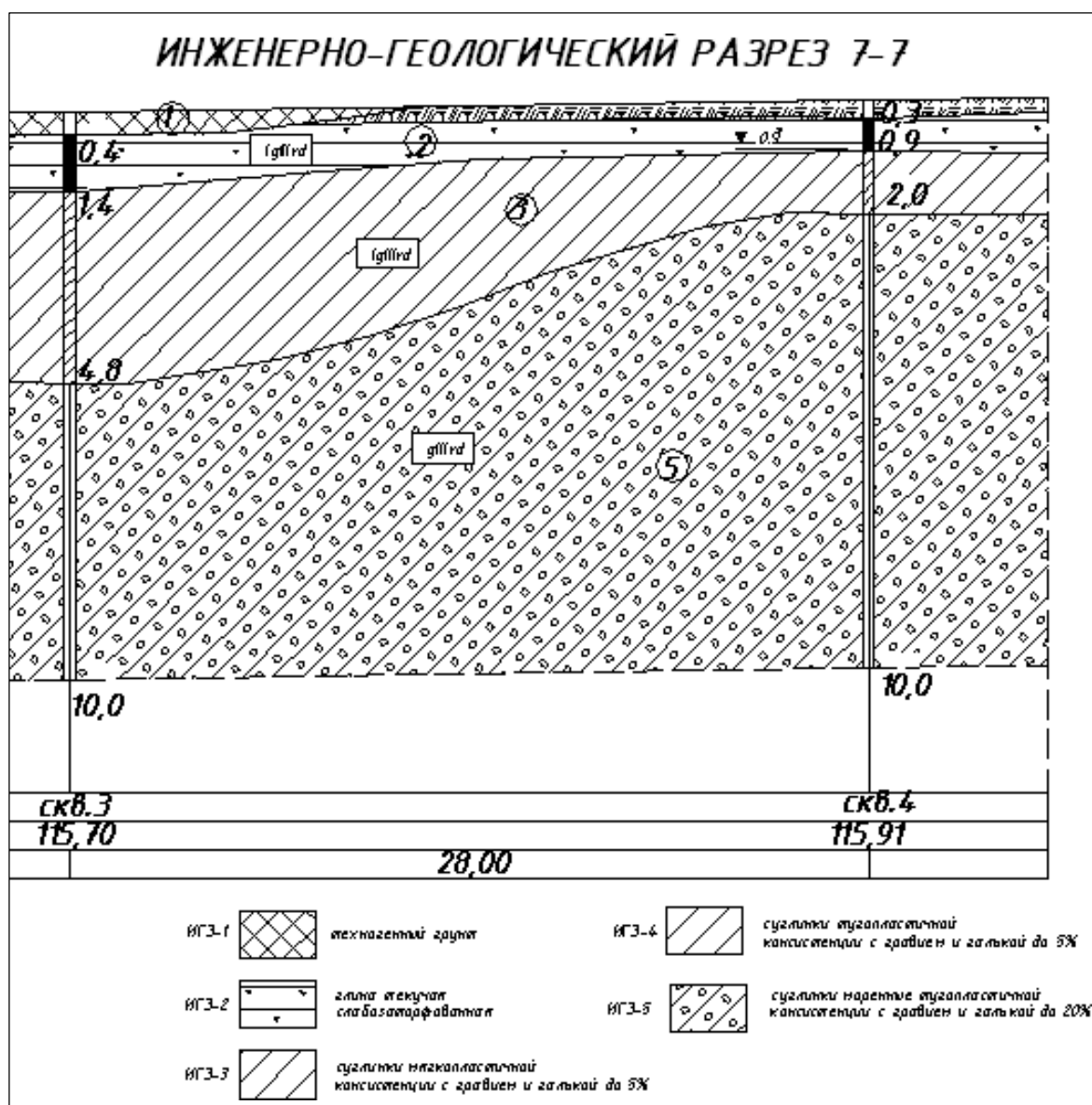
Инженерно-геологический разрез 7-7
