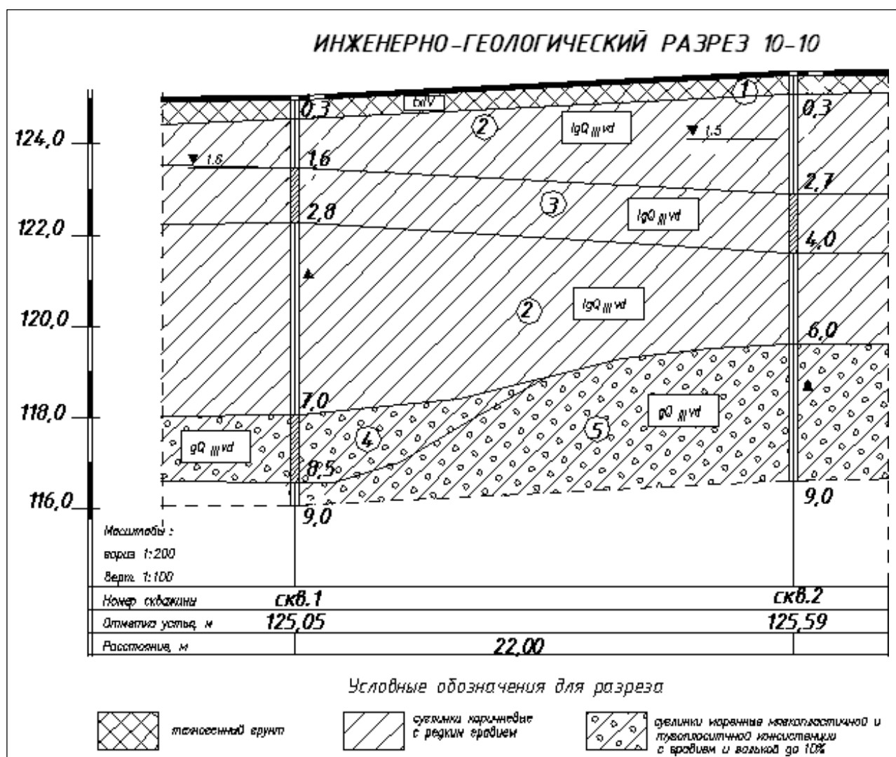
Инженерно-геологический разрез 10-10
