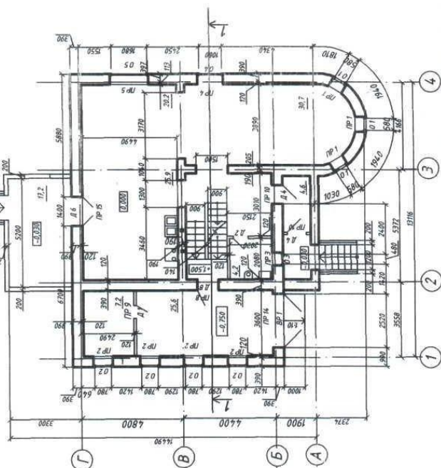
ПЛАН 1 ЭТАЖА
