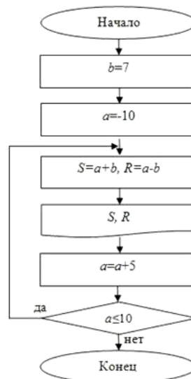
Рис. 1. ... алгоритм
