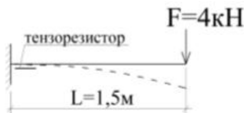
Рис. 1 Расчетная схема натурального испытания
