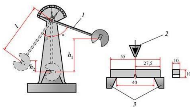
Рисунок 1. Схема испытаний на ударный изгиб: 1 - маятниковый копер; 2 - нож маятника; 3 – опоры с установленным на них образцом
