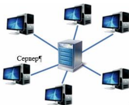
Рисунок 4 – Топология типа ...
