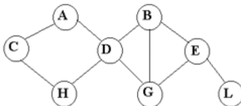
Рисунок 1 – ...модель данных
