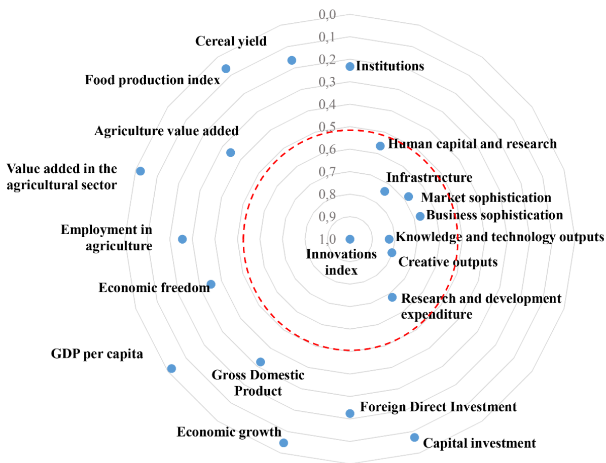
Рисунок 4 – Солнечная диаграмма матрицы корреляции [составлено автором]
